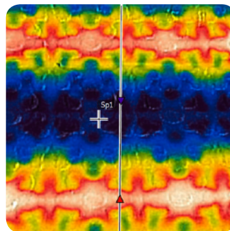
IMAGEN TERMAL DEL FLEXBONE® HEAT
